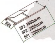
Trapdoor Platforms (OP3/OP2/OP1) 开窗平台板
