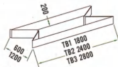
Toeboard Sets (TB1/TB2/TB3) 踢脚板
