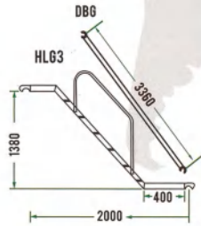
(HLG3/DBG) 三级架斜跨梯
