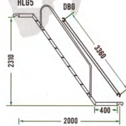
(HLG5/DBG) 五级架斜跨梯
