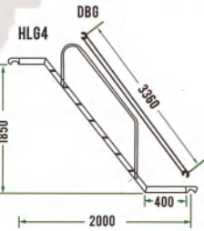
(HLG4/DBG) 四级架斜跨梯
